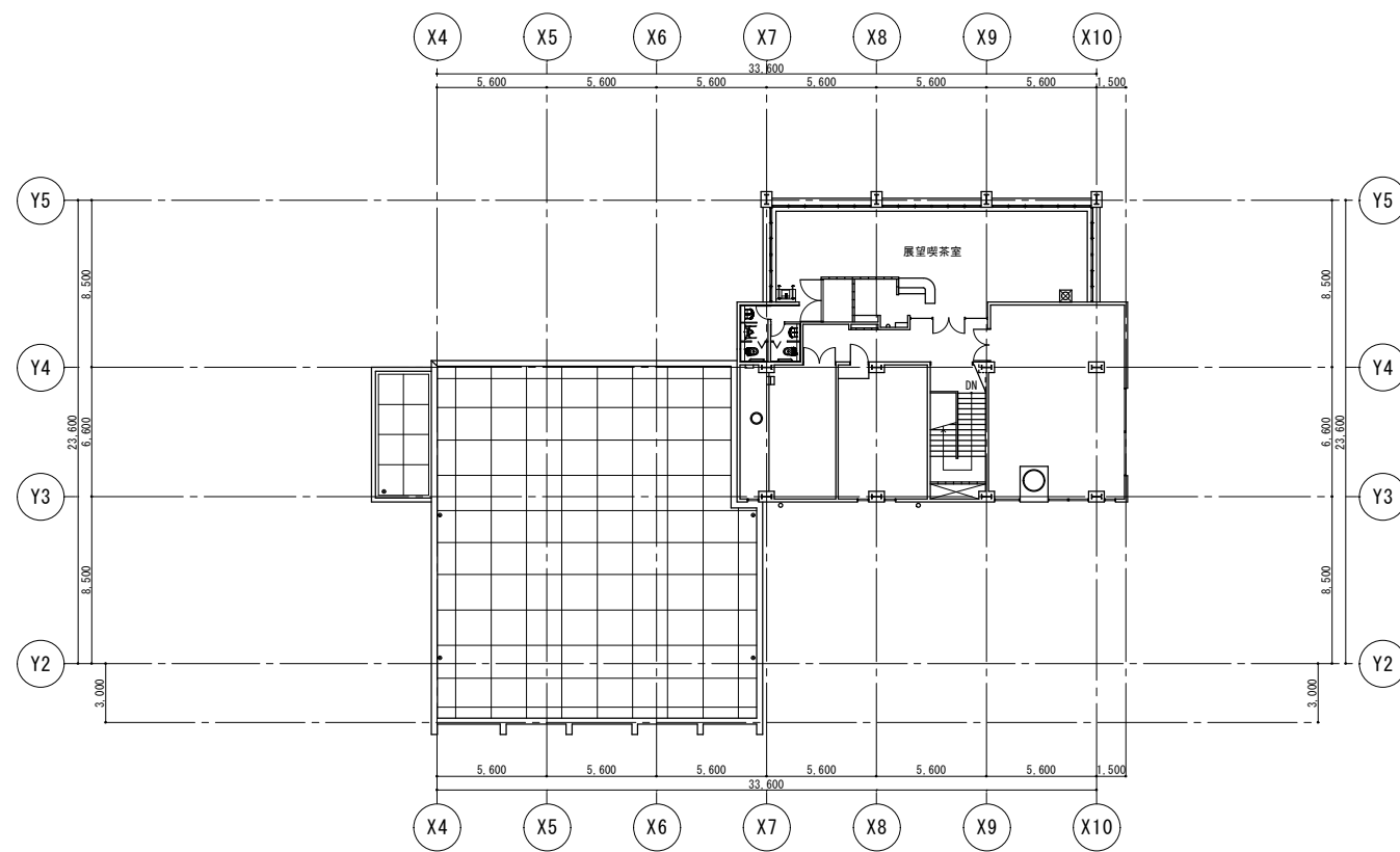
塔屋 2 階平面図
